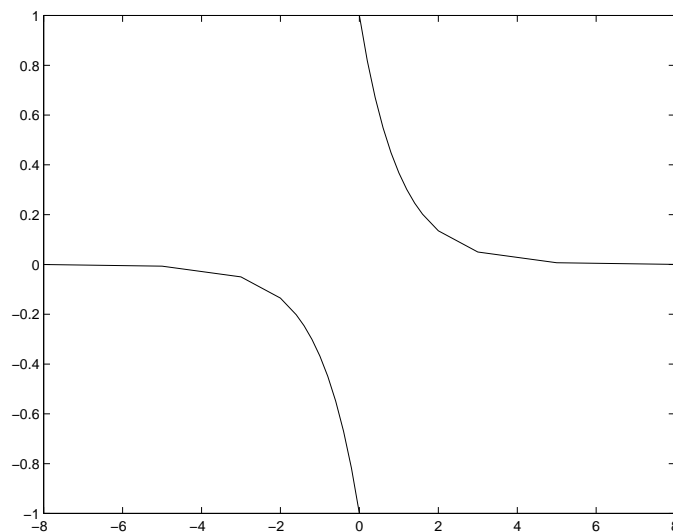
Réponse impulsionnelle du filtre de dérivée.
